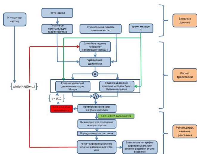
Рис. 1 Блок-схема программы
